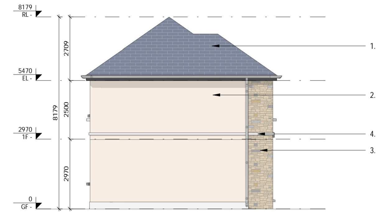
4 Elevation 04 1:100
