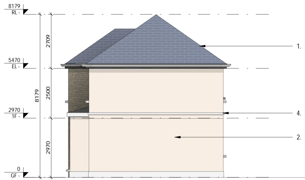
2 Elevation 02 1:100
